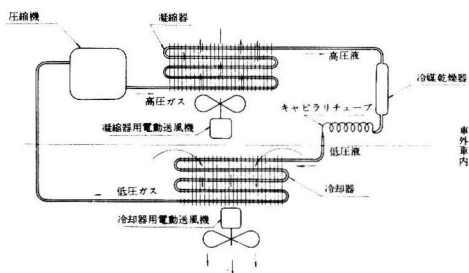
冷凍サイクルの例
