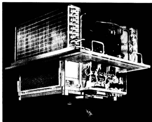
写真-2 特急形電車・気動車の天井形分散ユニットクーラ外観
