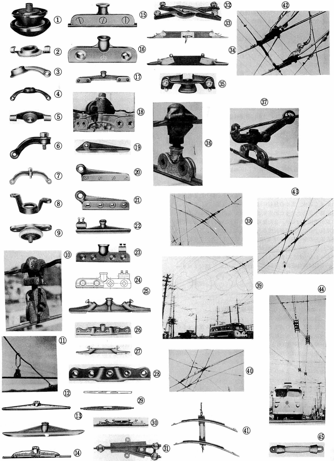
架線金具のいろいろ
