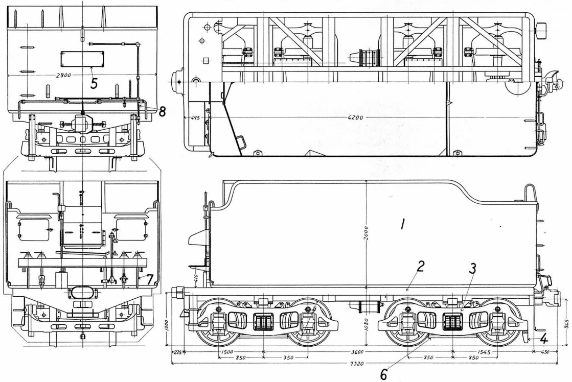
舟底形炭水車
