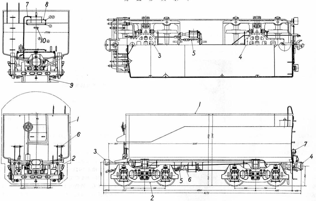
舟底形炭水車
