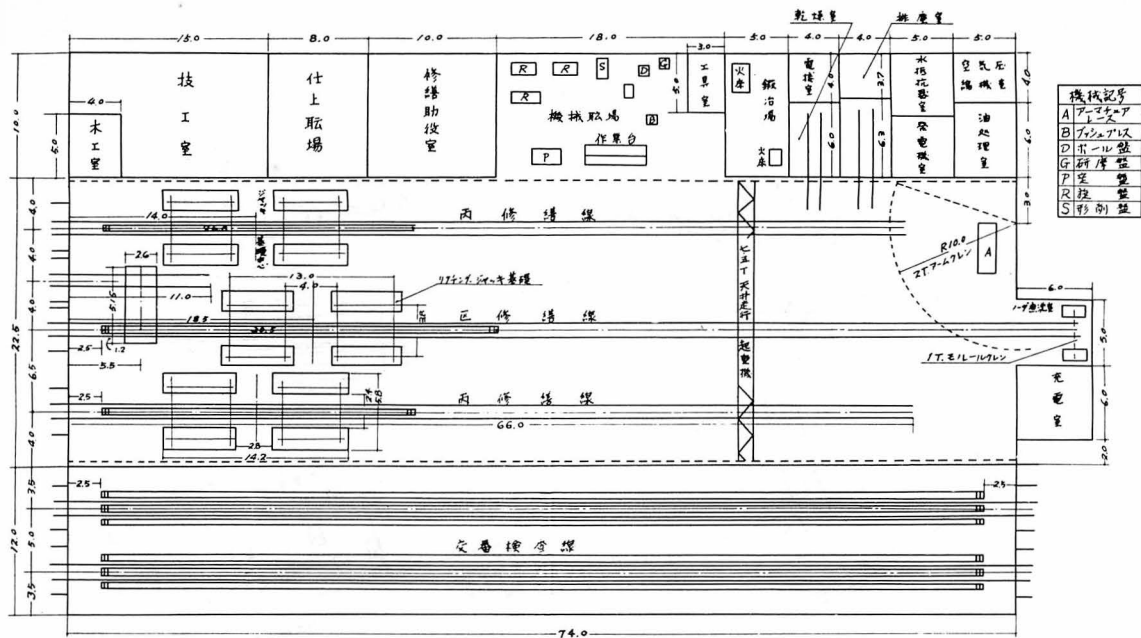
3. 電気機関車検修車庫 (その1)
