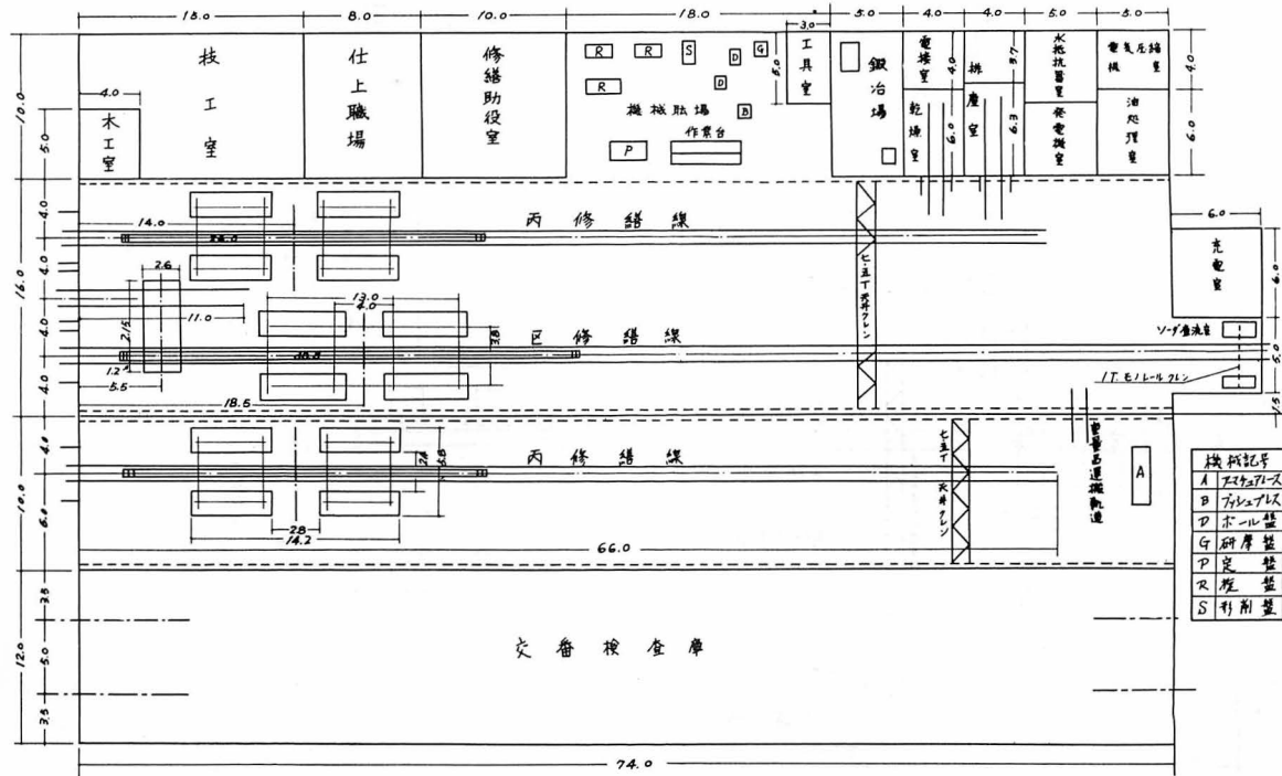
4. 電気機関車検修車庫 (その2)
