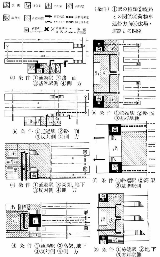
駅本屋一般計画
