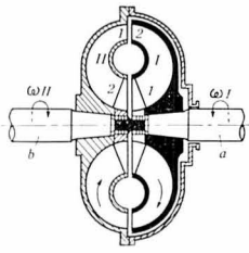
1. 液体・継手
