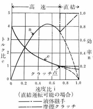
5. 液体変速機特性曲線
