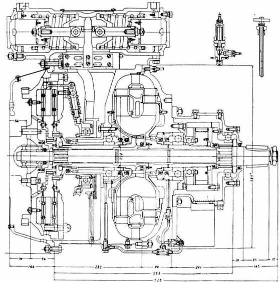
6. リスホルム・スミス形液体変速機
