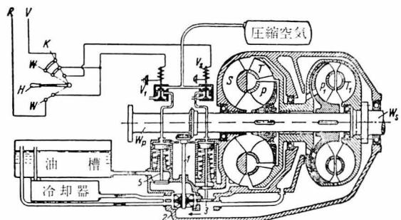
8. ホイト形液体変速機
