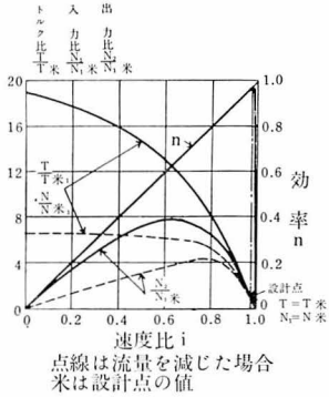
2. 液体継手性能曲線
