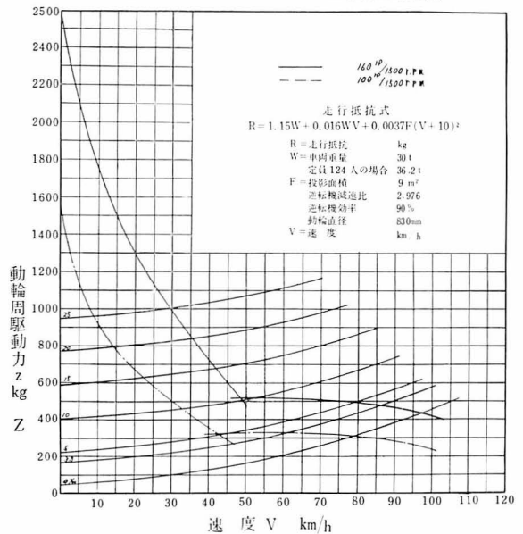
7. キハ44500形ディーゼル動車特性曲線
