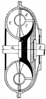
3. 液体変速機
